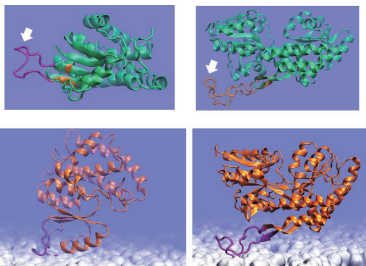
図4 接着ループを移植したタンパク質の接着 MD の結果
