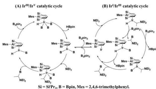
Scheme 1. Ir(III) aluminabenzenes 錯体による sp 3 CH 結合のボリル化反応の可能な反応機構
