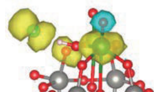
図2. 触媒-塩化物イオン複合体のスピン密度分布
