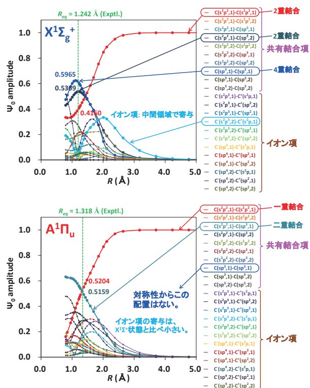
図 5. C_2 分子の C-C 化学結合の解析 化学フォーミュラ理論に基づく波動関数の amplitude
