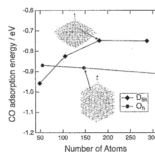
図 1. 各 NP 構造への CO 吸着エネルギー
