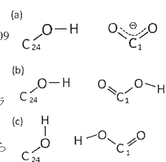
図 1 注目した部位における水素結合の状態 (a) プロトンなし (b) プロトンあり I (c) プロトンあり II
