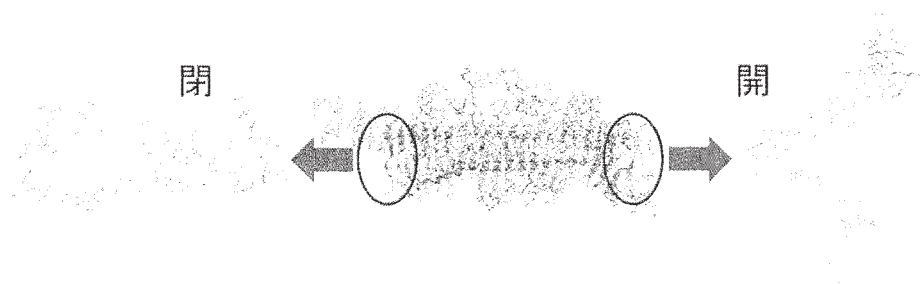
図1 水中における A \beta アミロイド線維の両末端の構造。
