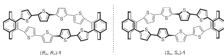
図1 化合物 1 の構造
