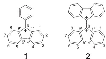
図 1. フルオレニルカチオン
