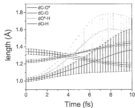
図 2: \text{H}_2\text{CO}_3 の OH, CO 結合の時間変化。*は励起原子を示す。
