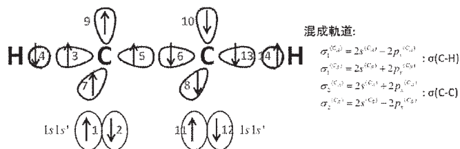
図 4. C 2 H 2 分子の初期関数と電子配置
