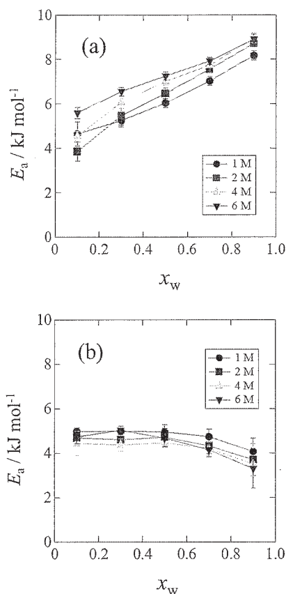
図2. (a)水および(b)シクロヘキサンの拡散係数の活性化エネルギーの組成および密度に対する依存性。
