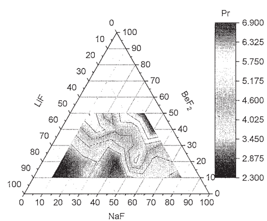
図 4 プラントル数評価結果 (1273 K)
