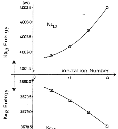
Fig.2 自由原子モデルでの価状態に対するCa K α , K β のシフト
