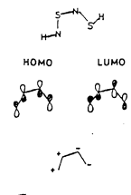
図6. HOMO, LUMO の位相
