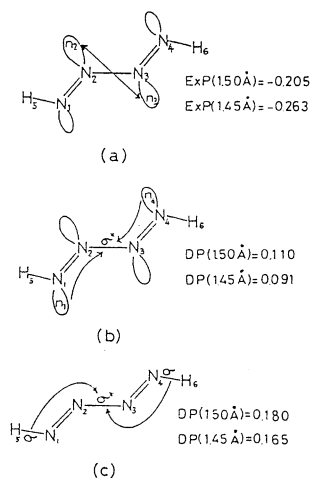
図2. 窒化水素の不安定化の因子
