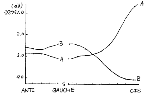
図1. 1,4-dithioglycol の S-C-C-S 二面角と、基底は \omega オール起状態のポテンシャル曲線
