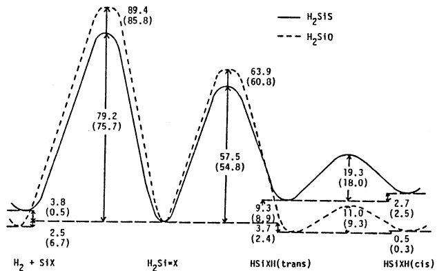
図5 零点補正した CI(SDQC)/6-31G**/16-31G 値 (kcal/mol)
