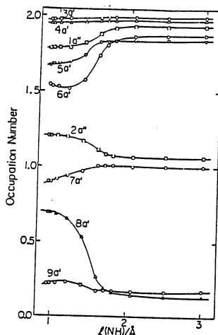
図4 軌道占有数の変化 (HNO, \text{\AA}^\circ , STO3G, CASSCF)
