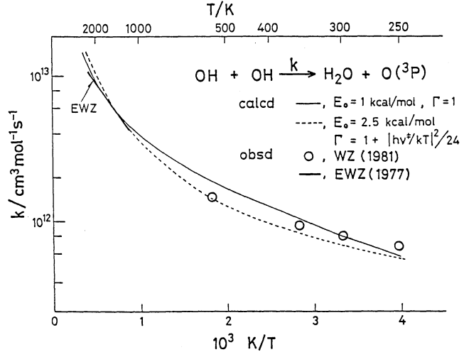
図6. OH + OH → H 2 O + O(3P) の2次反応速度定数 k のアレニウスプロット。
