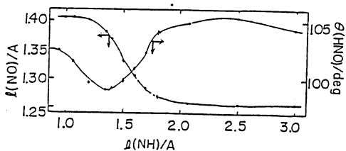
図3 HNO ( \text{\AA}^\circ ) の分子の形
