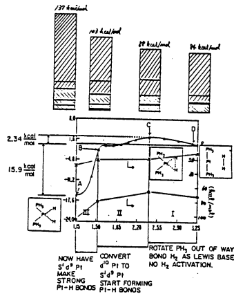
図6. Pt(PH 3 ) 2 + H 2 の反応経路上の Pt-H 結合の d 電子エネルギーの解析
