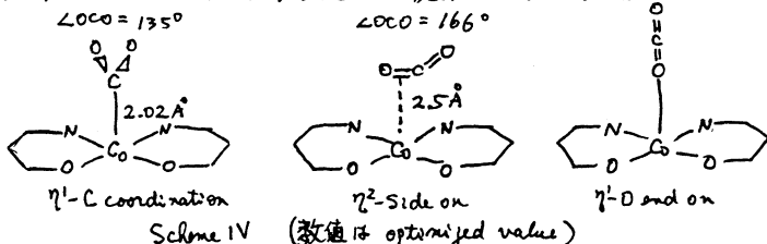
Scheme IV (数値は optimized value)
