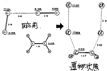
図6 (Cl 2 ) 2 + H 2 C=CH 2 付加反応。
