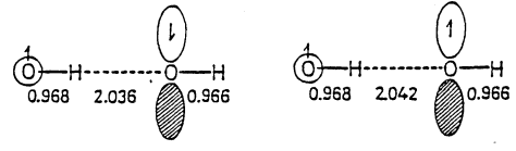
図5. 水素結合によるOH 2量体の構造。
