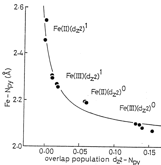
図2. FeP(py) 2 錯体におけるFe-Npy結合距離と d_{z^2} -Npy overlap populationの相関グラフ。 (d_{z^2})^1 、 (d_{z^2})^0 は d_{z^2} 軌道の占有電子数を表わす。
