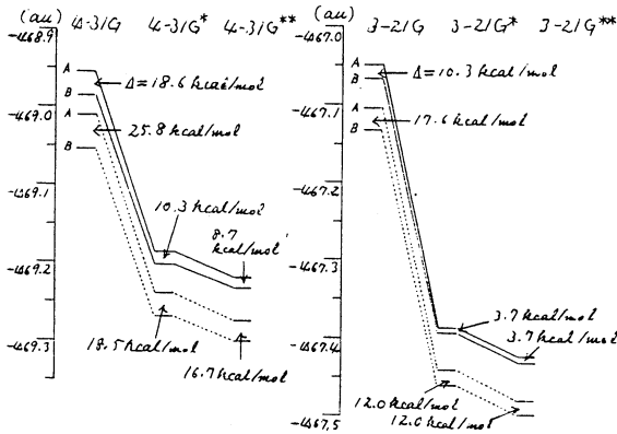
図2 トリプトシン遷移状態のエネルギー A: 図1 a. に相当, B: 図1 b. に相当. 実線: 孤立系, 破線: 酵素の静電場中.
