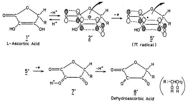
図 8 ビタミン C の 2 電子酸化過程
