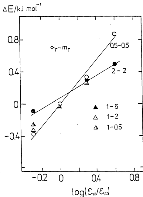
図6 拡散の活性化エネルギー差 \Delta E の \epsilon 依存性
