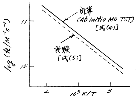
図 2. \text{HN}_3 への H 付加速度定数
