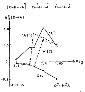
図13 RによるD→Aの負電荷の移動
