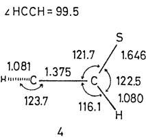
図 4 4 の平衡構造
