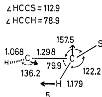
図 5 遷移状態の構造
