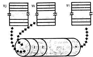
図1 パイプライン方式のベクタプロセッサの演算処理。ベクタV j とV k の加算が連続的に行われ結果がV i に入れられる。
