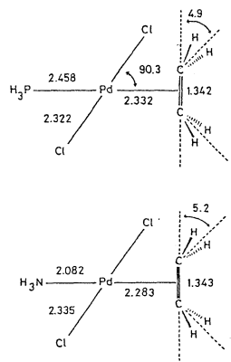
図14. [\text{Pd}(\text{C}_2\text{H}_4)_2\text{Cl}_2\text{X}] の構造
