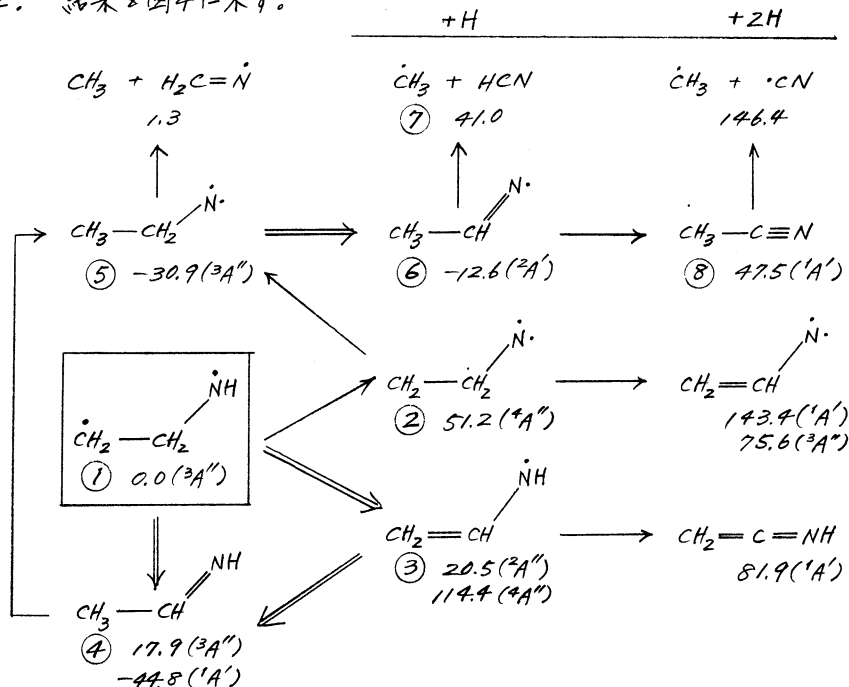
図4 \text{CH}_2\text{CH}_2\text{NH}(^3A'') のH移動および分解によるエネルギー変化
