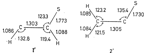
図 2. 励起状態 ( 1^1A' ) の平衡構造
