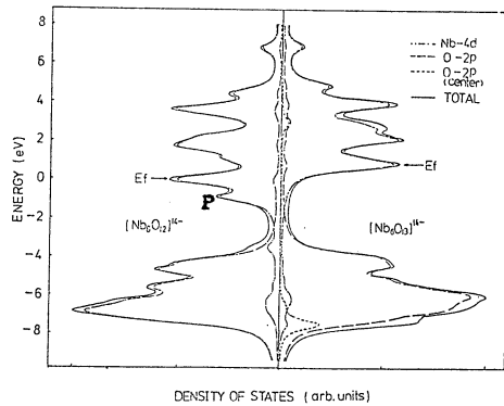
図4. 状態密度
