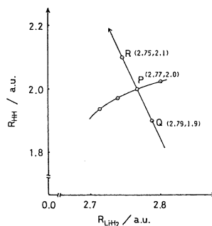
Fig. 7 反応座標上にとった点P, Q, R
